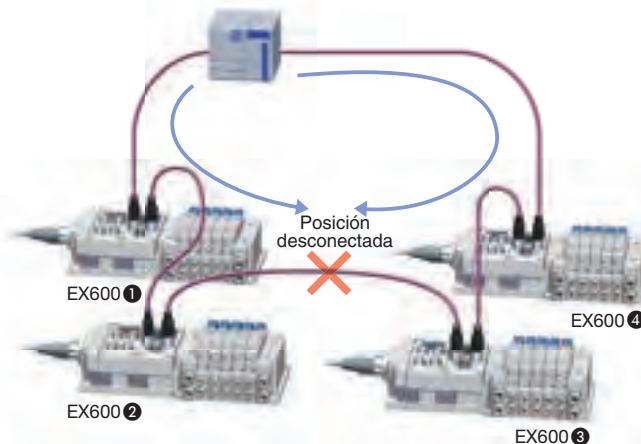
Flujo de datos cuando el cable de comunicación está desconectado
