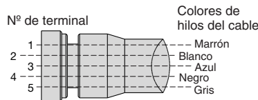
Conexiones
