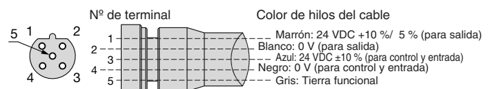
Conexiones
