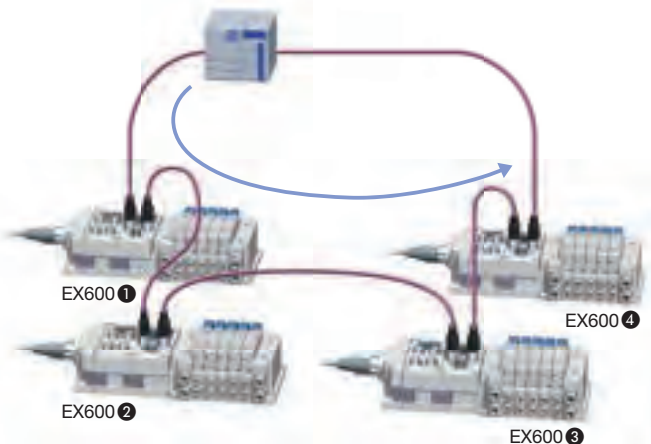
Flujo normal de datos
