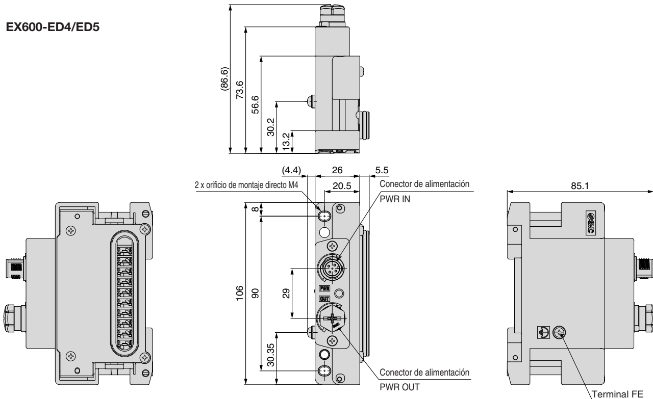
Conector de alimentación PWR OUT: conector M12, macho de 5 pins, código A
