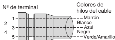
Conexiones
