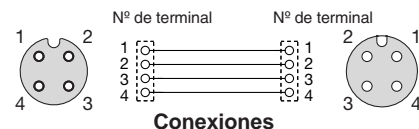
Conexiones
